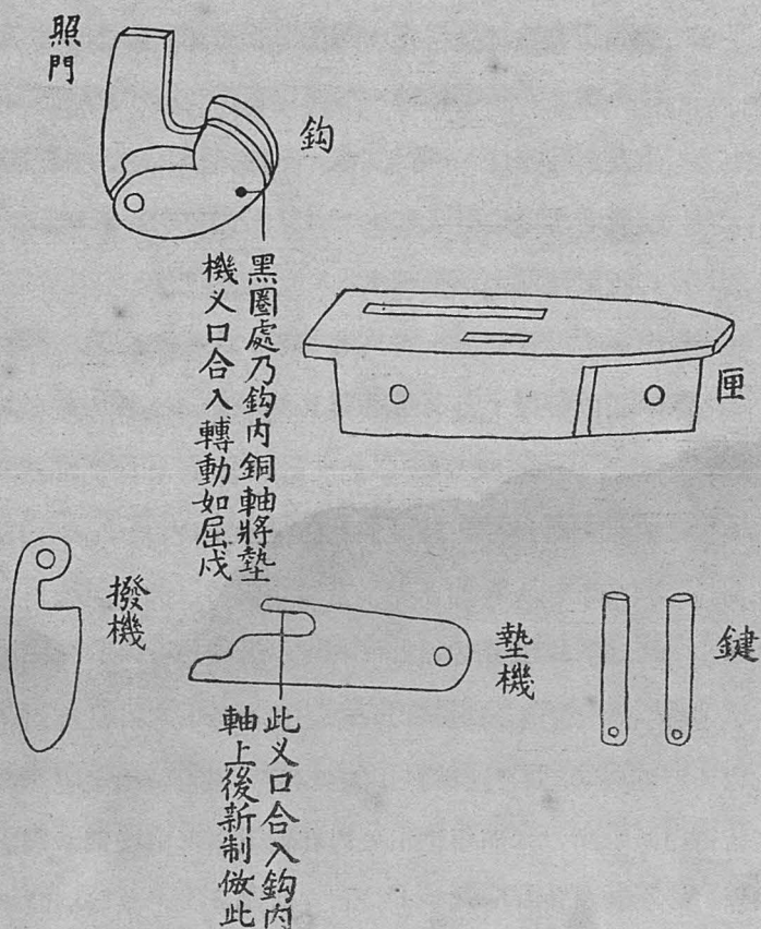
法古制銅弩機散圖
