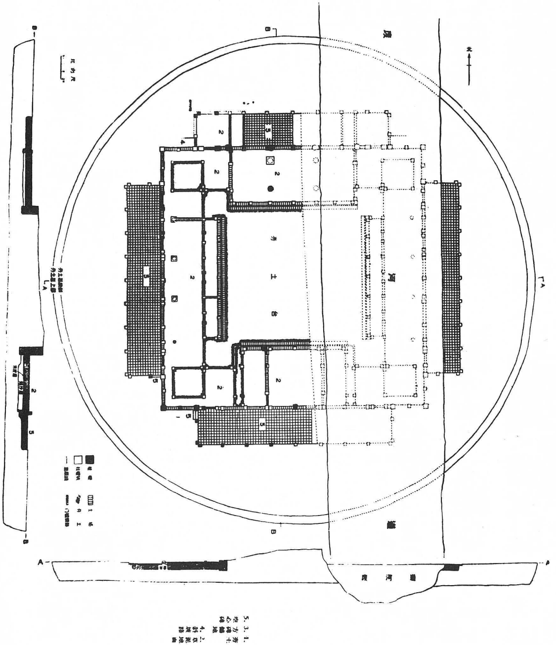
西安西郊漢代建築基址中心建築平剖面實測圖 (採自唐金裕西安西郊漢代建築遺址發掘報告)
