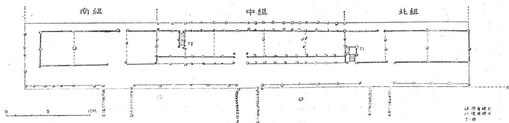
圖十 小屯乙八基址礎石的復原（《考古人類學刊》，39/40，頁144）
