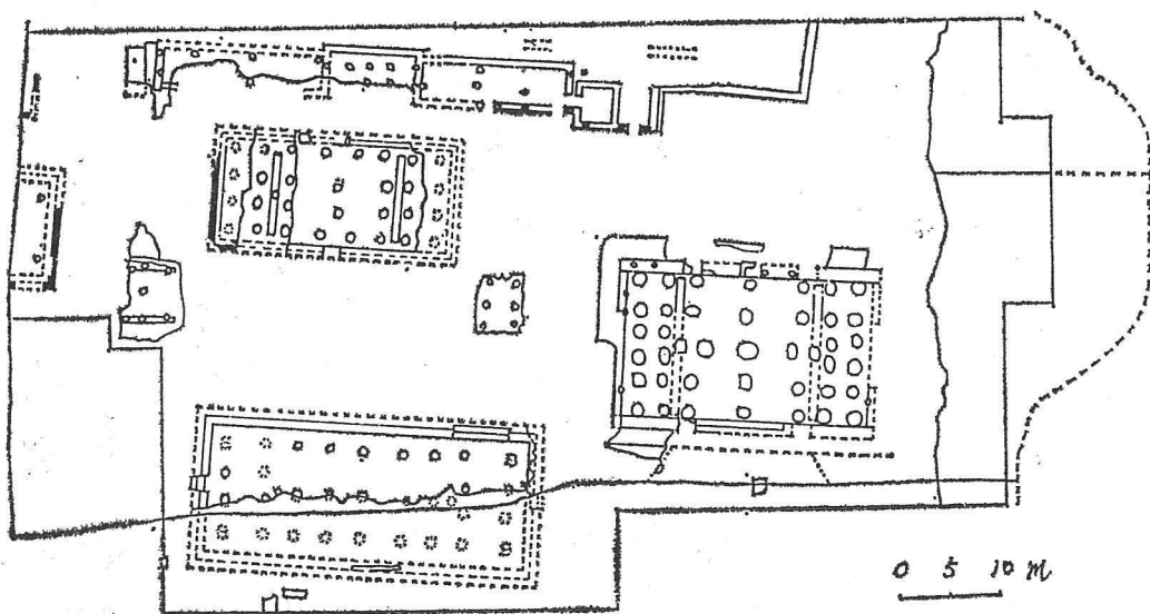
圖十一 召陳西周甲區廟宮羣平面圖（《文物》，1981年3期，頁12）
