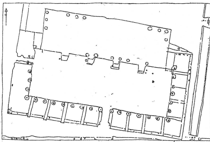
圖九 尸鄉溝商城 J1D4 廟宮基址平面圖（《考古》，1985年4期，頁326）
