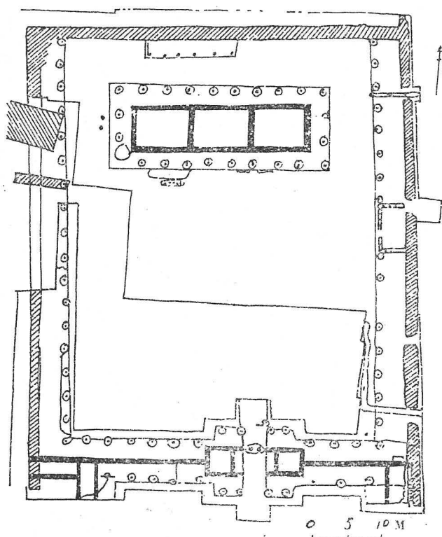
圖八 二里頭二號廟宮基址平面圖（《考古》，1983年3期，頁207）
