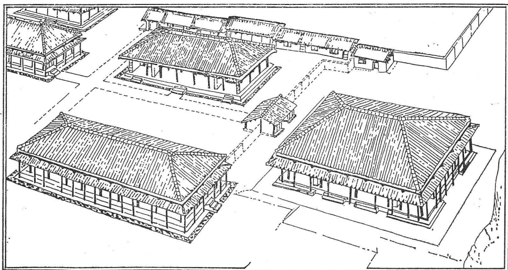
圖十二 召陳甲區廟宮羣外觀示意圖（據《文物》，1981年3期，頁41重繪）
