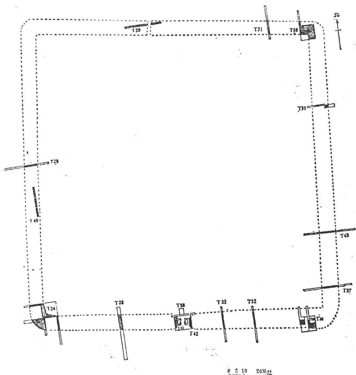
圖三 平糧臺古城垣探測圖（《文物》，1983年3期，頁27）
