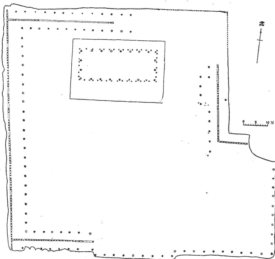
圖七 二里頭一號廟宮基址平面圖（《考古》，1974年4期，頁235）
