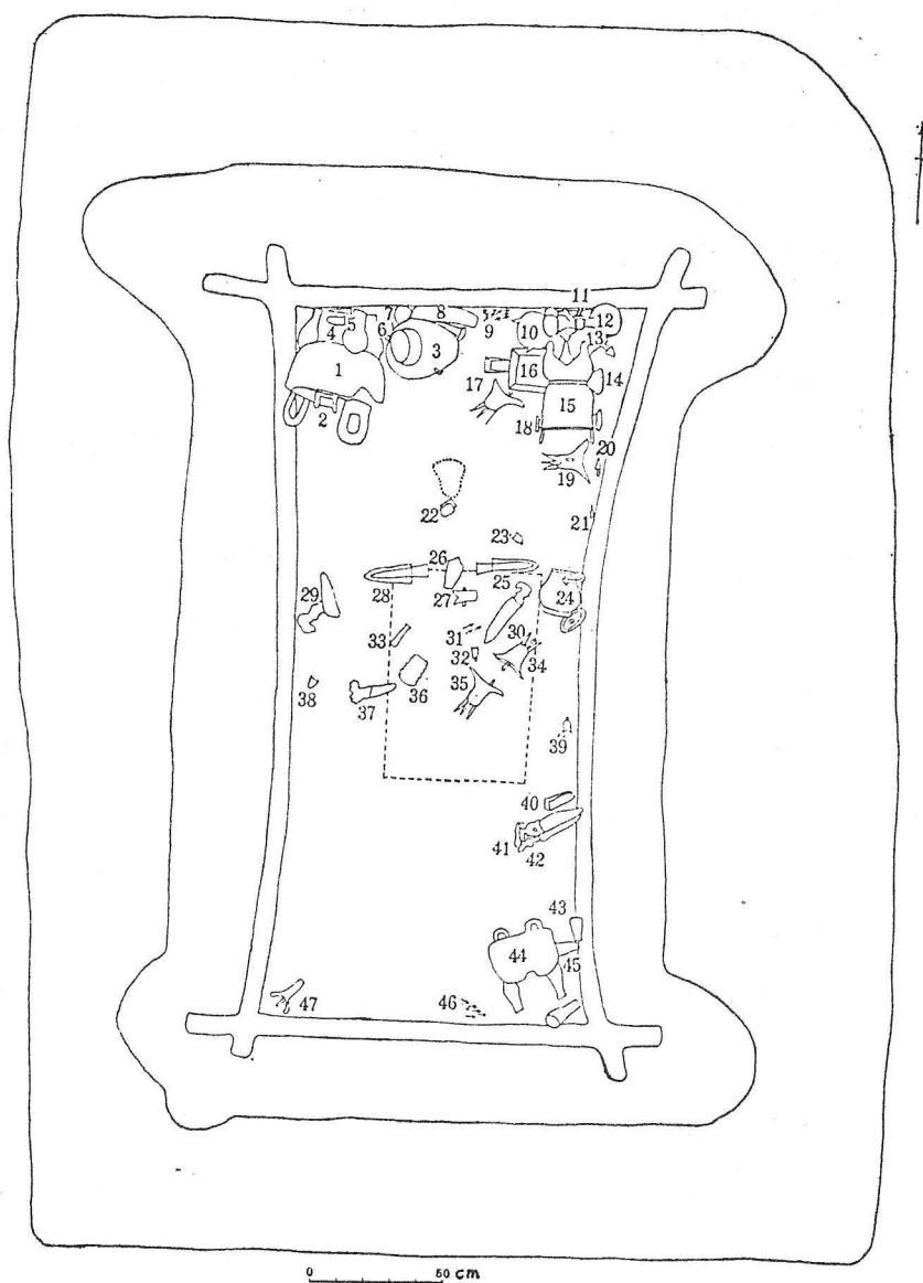
圖十九 羅山嶺張79M 1 平面圖（考古》1981年2期，頁112）
