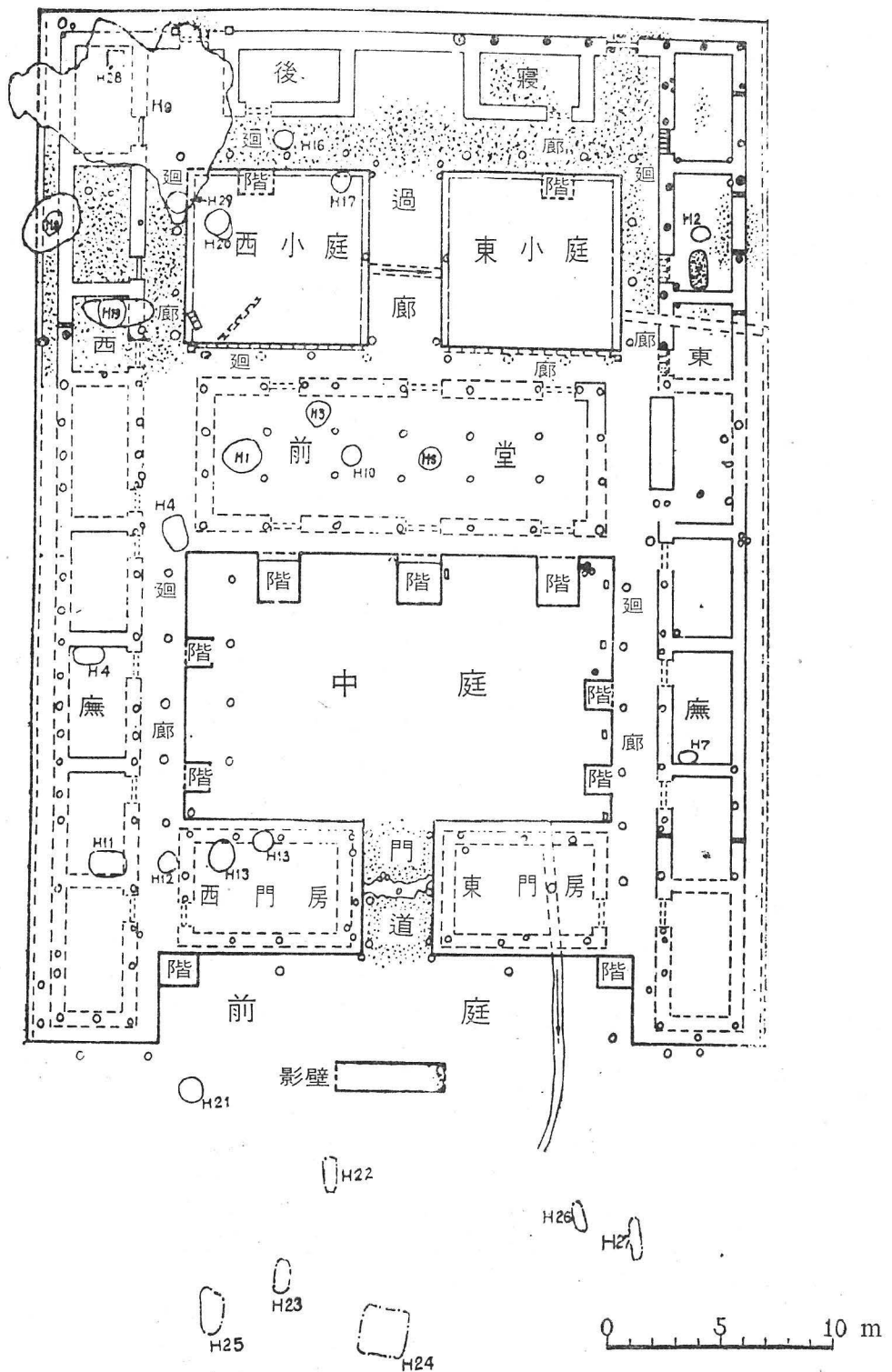
圖六 鳳雛西周甲組建築基址平面圖(《文物》, 1979年10期, 頁29)
