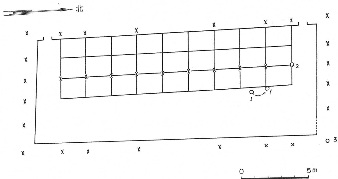
圖三：甲十三基址礎石及內部結構復原示意圖
